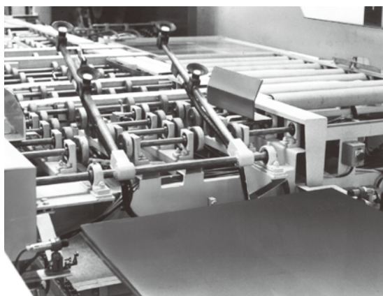
翻 转 机
