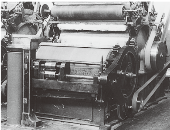
梳绵机
