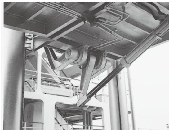
渡船用舷梯
