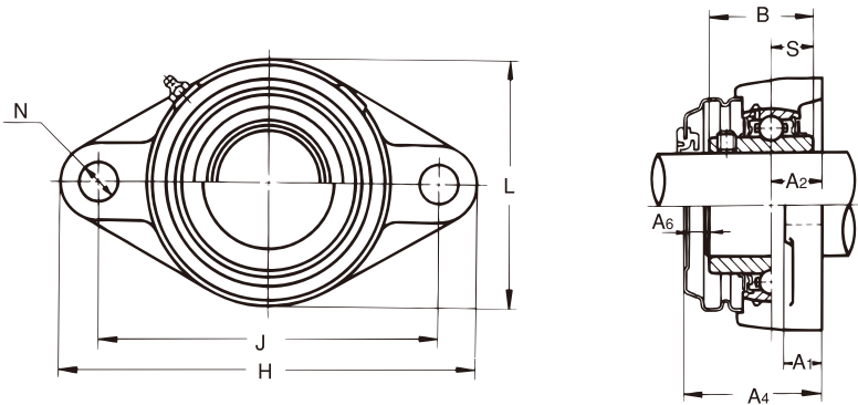
带不锈钢板制防护盖
