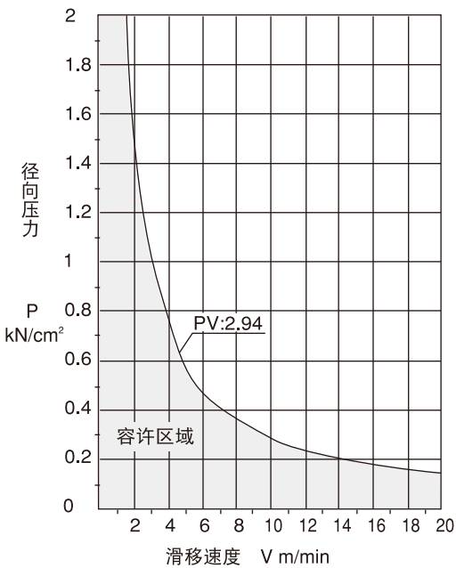
<图5.3> 关节轴承的容许PV值
