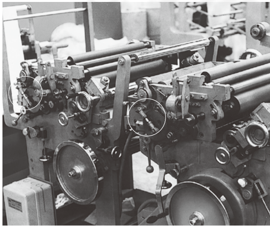
印刷机械
