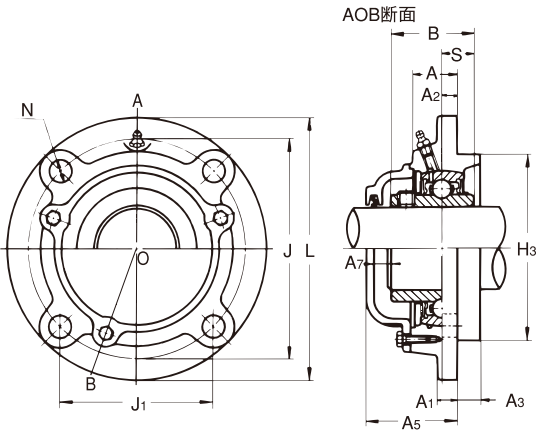
带铸铁制防护盖
