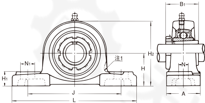
注1是表示UCPX00型的形状。
