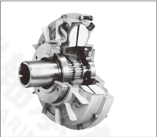
液力偶合器
