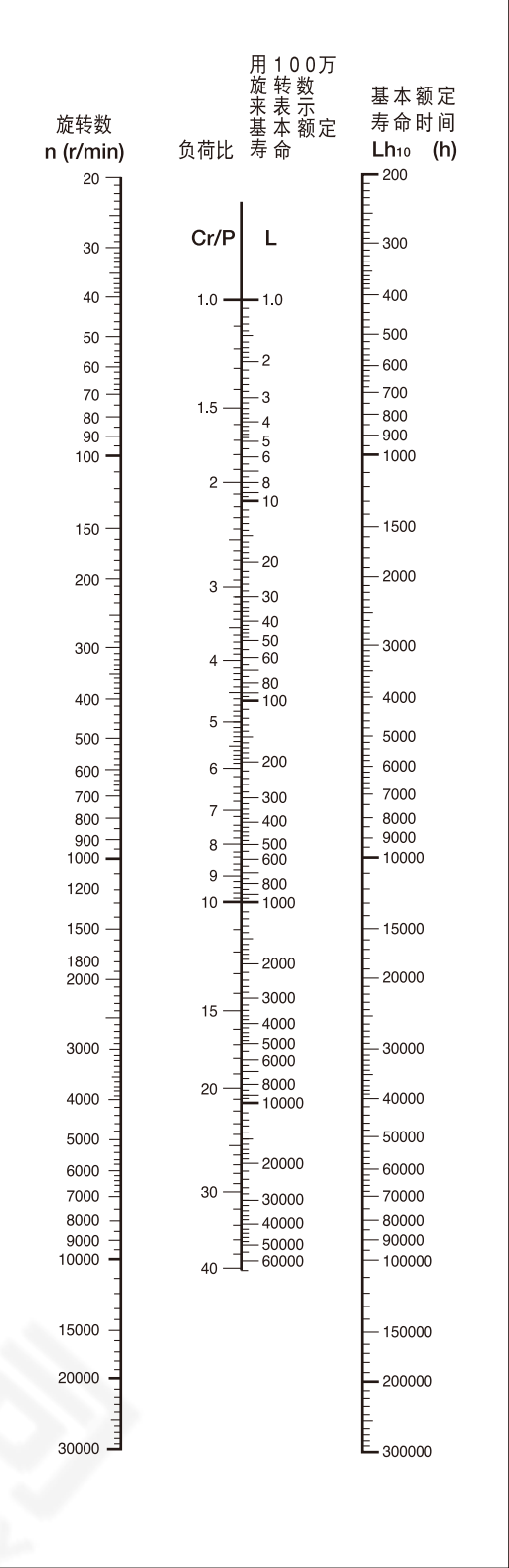
<图4. 5> n-Cr/P-L_{h10} 计算图表
