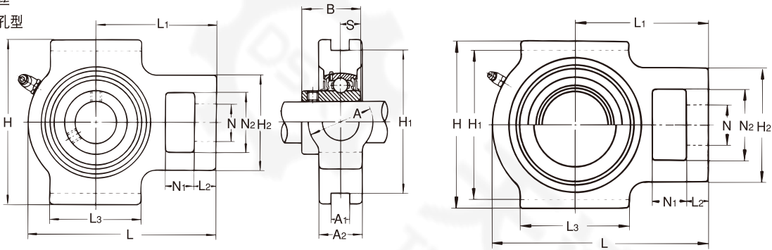
带钢板制防护盖
