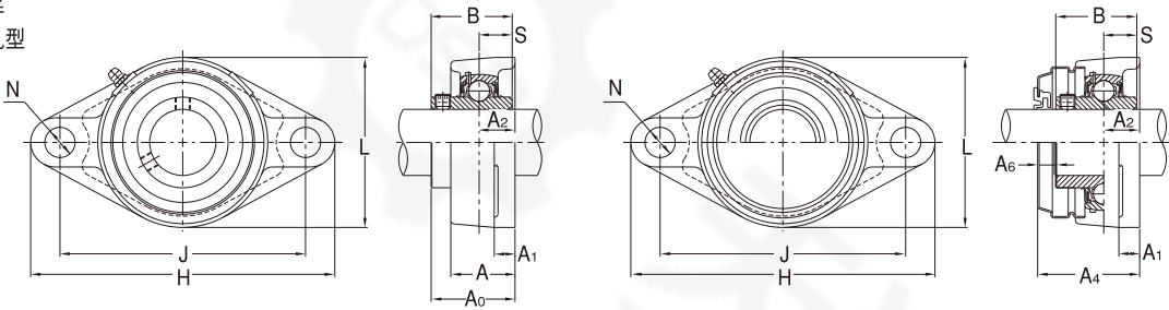
带不锈钢钢板制防护盖
