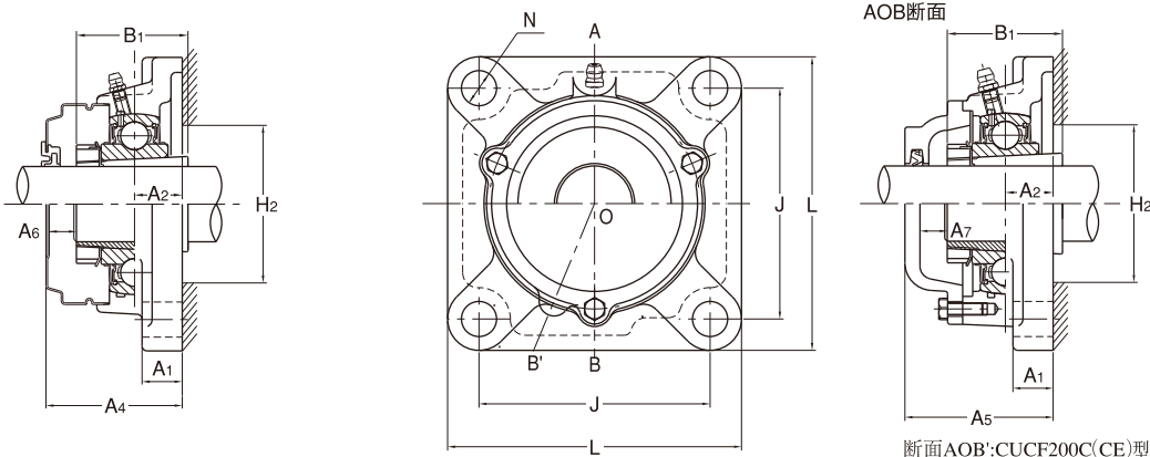
带铸铁制防护盖
