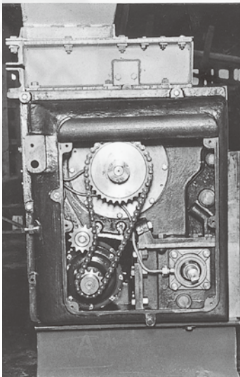
加煤机
