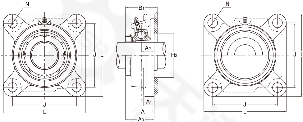
带钢板制防护盖
