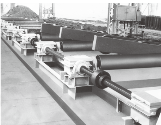
滚筒同轴插口
