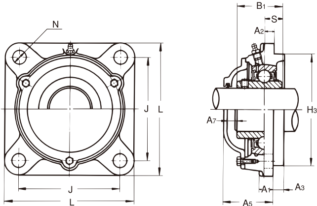
带铸铁制防护盖
