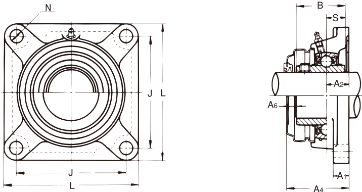
带不锈钢钢板制防护盖
