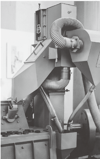
集尘器
