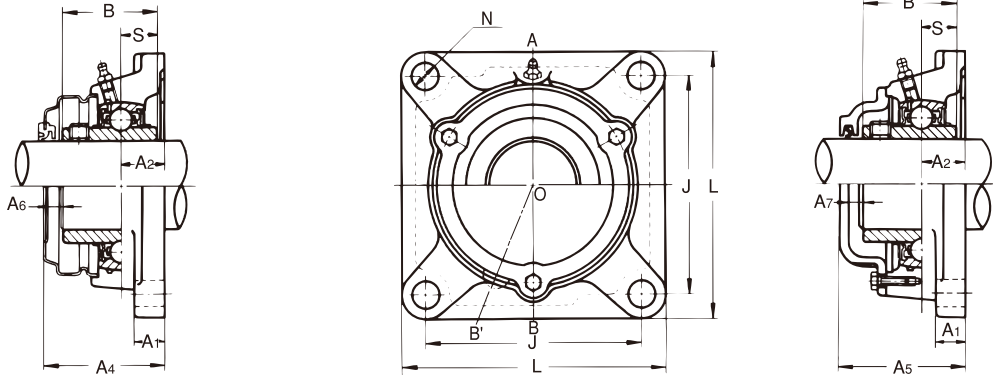
带铸铁制防护盖
