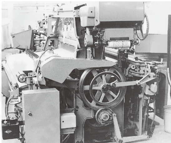
编织机
