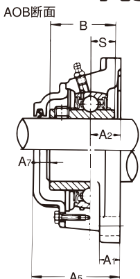
断面AOB':CUCF200C(CE)型 断面AOB :CUCF300C(CE)型
